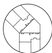
45° stolpeløsning Træ (Udvendig)
