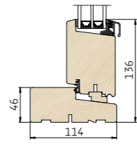
2 Lodret snit i bundkarm/spændestykke
