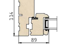
4 Vandret snit i sidekarm/ramme
