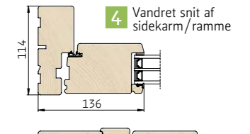
4 Vandret snit af sidekarm/ramme
