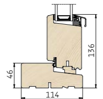
2 Lodret snit i bundkarm/spændestykke
