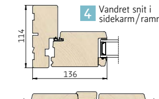
4 Vandret snit i sidekarm/ramme
