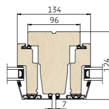
4 Vandret snit i lodpost/rammer
