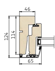
4 Vandret snit i sidekarm/ramme
