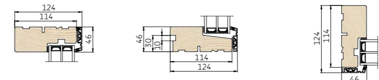
1 Lodret snit i overkarm 2 Lodret snit i bundkarm 3 Vandret snit i sidekarm
