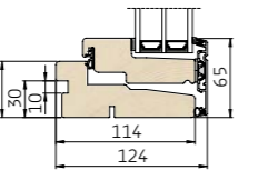
2 Lodret snit i bundkarm
