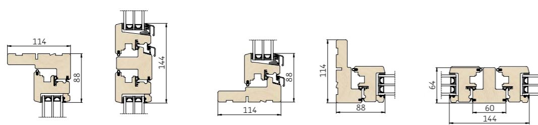
1 Lodret snit i overkarm/ramme 2 Lodret snit i tværpost/rammer 3 Lodret snit i bundkarm/ramme 4 Vandret snit i sidekarm/ramme 5 Vandret snit i lodpost/rammer Kan ikke leveres med bundpladenot pga. konstruktionen.
