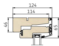
1 Lodret snit i overkarm/ramme
