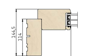
3 Vandret snit i sidekarm/ramme
