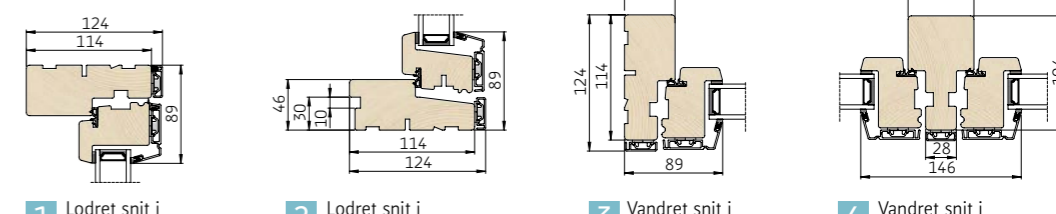
1 Lodret snit i overkarm/ramme 2 Lodret snit i bundkarm/ramme 3 Vandret snit i sidekarm/ramme 4 Vandret snit i lodpost/rammer
