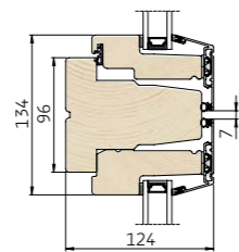
2 Lodret snit i vandret post/rammer
