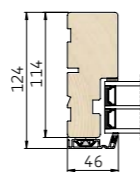
3 Vandret snit i sidekarm
