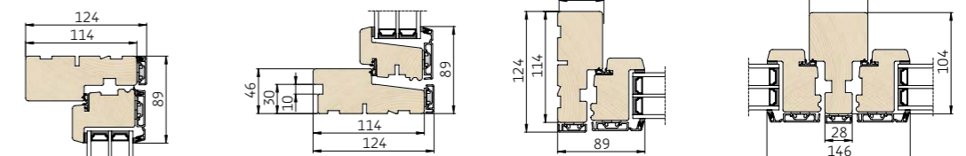
1 Lodret snit i overkarm/ramme 2 Lodret snit i bundkarm/ramme 3 Vandret snit i sidekarm/ramme 4 Vandret snit i lodpost/rammer
