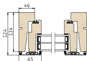
3 Vandret snit i sidekarme/rammer
