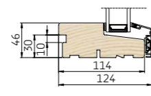
2 Lodret snit i bundkarm
