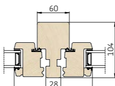
4 Vandret snit i lodpost/rammer
