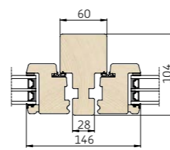
4 Vandret snit i lodpost/rammer
