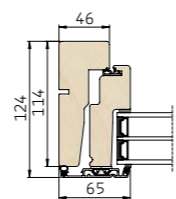
4 Vandret snit i sidekarm/ramme
