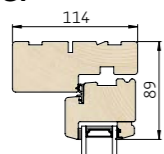
1 Lodret snit i overkarm/ramme
