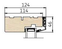
1 Lodret snit i overkarm
