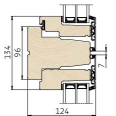
2 Lodret snit i vandret post/rammer
