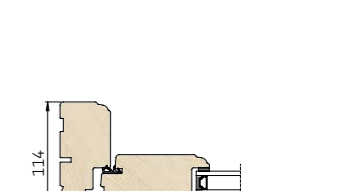
4 Vandret snit i sidekarm/ramme
