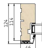
3 Vandret snit i sidekarm
