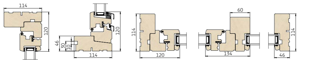
1 Lodret snit i overkarm/ramme 2 Lodret snit i bundkarm/ramme 3 Vandret snit i sidekarm/ramme 4 Vandret snit i lodpost/ramme 5 Vandret snit i sidekarm Alle elementer leveres med bundpladenot i som standard.
