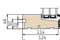
2 Lodret snit i bundkarm
