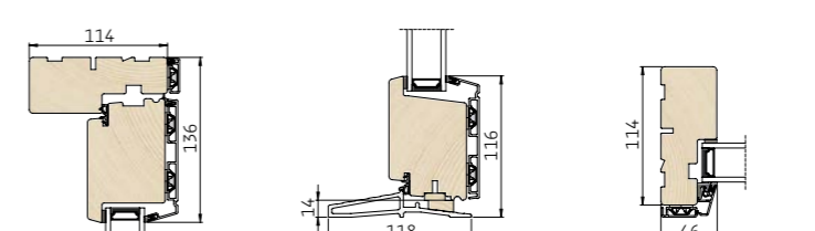
1 Lodret snit i overkarm/spændestykke 2 Lodret snit i bundkarm/spændestykke 3 Vandret snit i sidekarm
