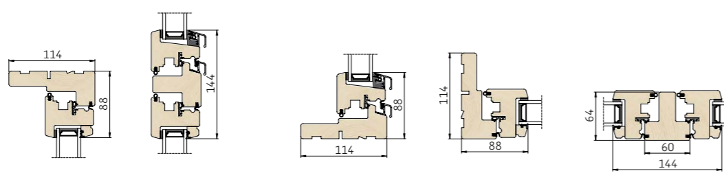
1 Lodret snit i overkarm/ramme 2 Lodret snit i tværpst/rammer 3 Lodret snit i bundkarm/ramme 4 Vandret snit i sidekarm/ramme 5 Vandret snit i lodpost/rammer Kan ikke leveres med bundpladenot pga. konstruktionen.
