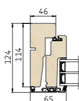
3 Vandret snit i sidekarm/ramme
