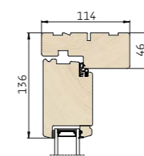
1 Lodret snit i overkarm/ramme
