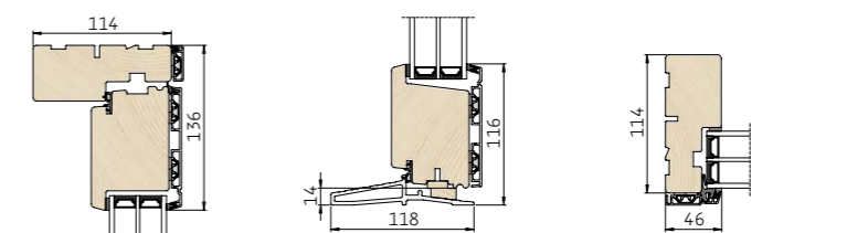
1 Lodret snit i overkarm/spændestykke 2 Lodret snit i bundkarm/spændestykke 3 Vandret snit i sidekarm
