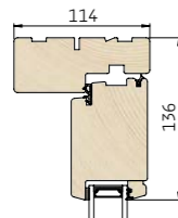
1 Lodret snit i overkarm/spændestykke
