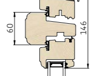
2 Lodret snit i vandret post/rammer
