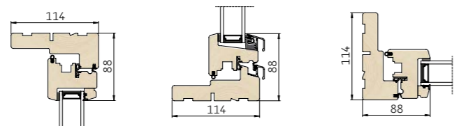
1 Lodret snit i overkarm/ramme 2 Lodret snit i bundkarm/ramme 3 Vandret snit i sidekarm/ramme Kan ikke leveres med bundpladenot pga. konstruktionen.
