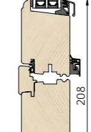
2 Lodret snit i midterrammer
