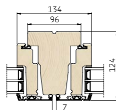
4 Vandret snit i lodpost/rammer
