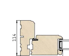
4 Vandret snit i sidekarm/ramme
