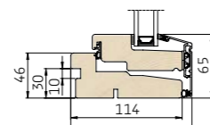
2 Lodret snit i bundkarm
