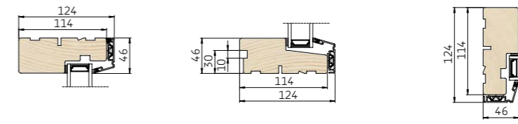
1 Lodret snit i overkarm 2 Lodret snit i bundkarm 3 Vandret snit i sidekarm
